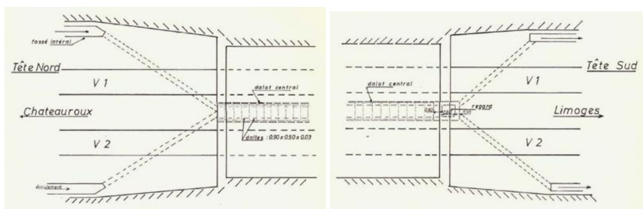
Plans vus de dessus de l'entrée et de la sortie du tunnel
