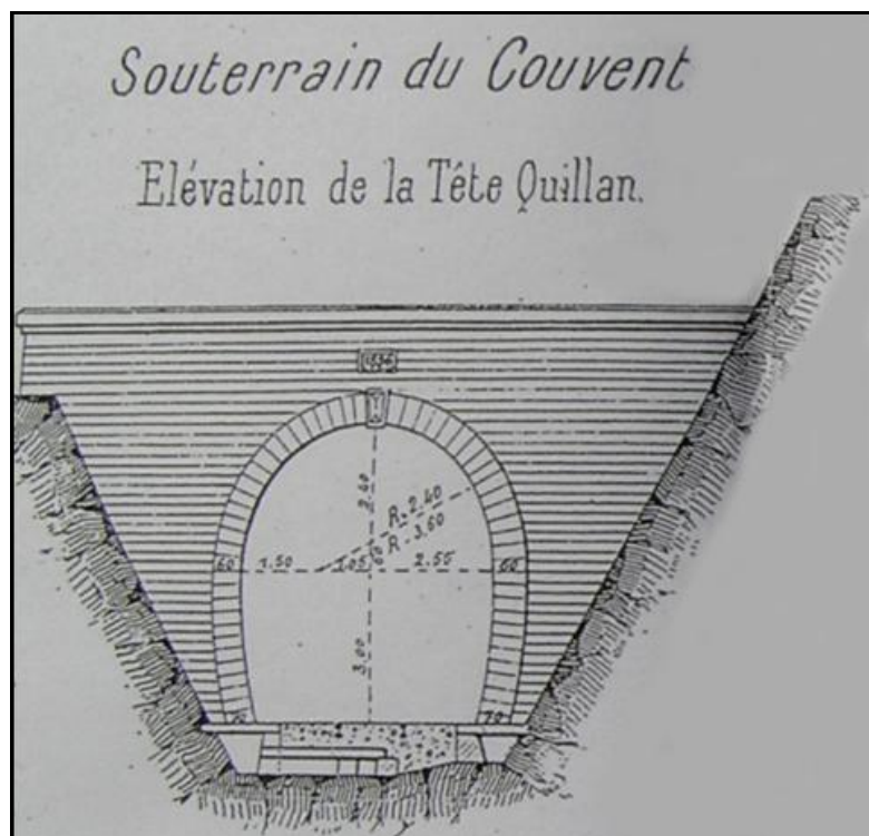
Plan du fronton d'entrée
